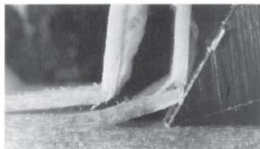
Фото 1: тип стружкообразования производит очень гладкую поверхность при резке параллельно с зерном.
